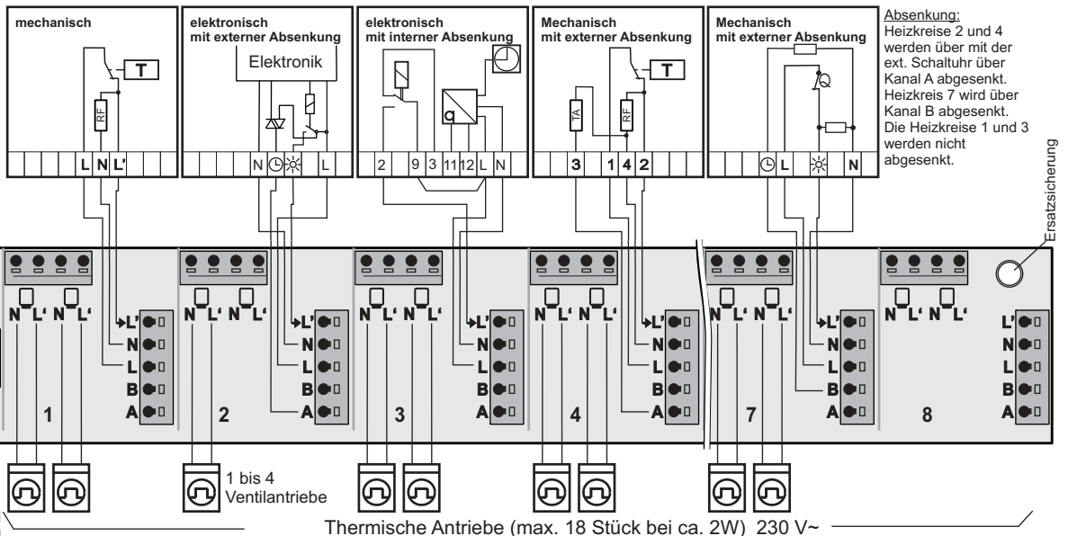
Raumtemperaturregler 230V~
