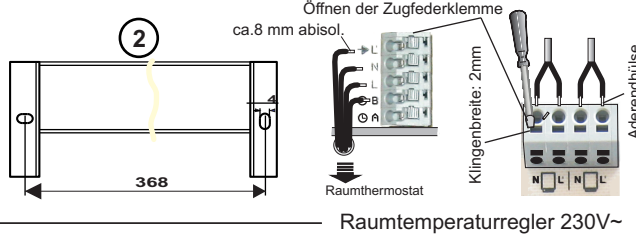
Raumtemperaturregler 230V~
